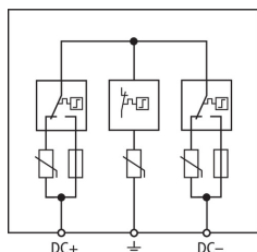
Kapcsolási rajz DCU YPV SCI 1000 1M
