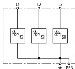
Kapcsolási rajz DSH TNC 255
