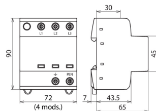
Beépítési méretek DSH TNC 255
