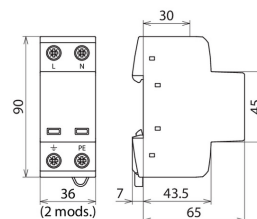
Beépítési méretek DSH TN 255
