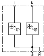
Kapcsolási rajz DSH TN 255
