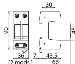
Beépítési méretek DG M TN 275
