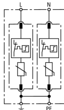
Kapcsolási rajz DG M TN 275
